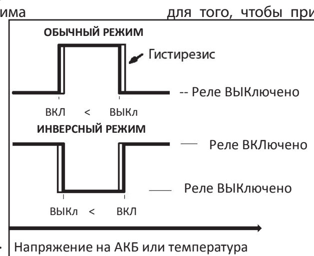
Рисунок 11. Режимы работы Реле
