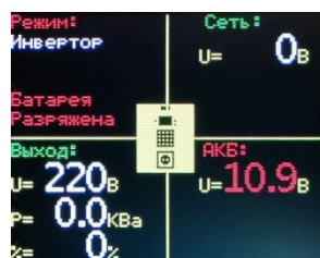
Рис.№4. Индикатор в режиме предупреждения.
